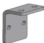
Endesbeslag 690434 1½" til mur 690433 2" til mur 690435 2" til spær 690435-01 2" til stolpe
