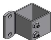
Enkelt inkl. rørbøjle 691200-08 2" 691200-098 1½"
